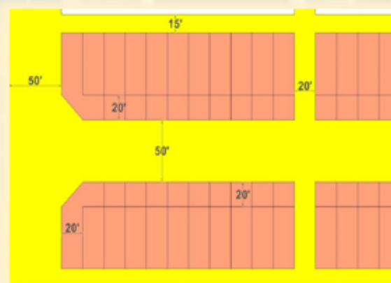
Ilustrasi ukuran lebar jalan dan anjakan bagi rumah teres kos rendah
